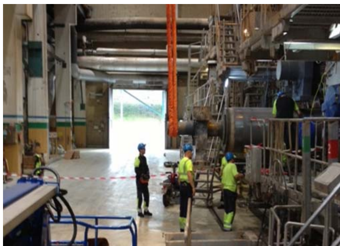
Här drar man ut valsen från maskinen
