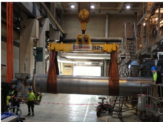
Här ser vi valsen ute från maskinen och nu ska den vändas.
