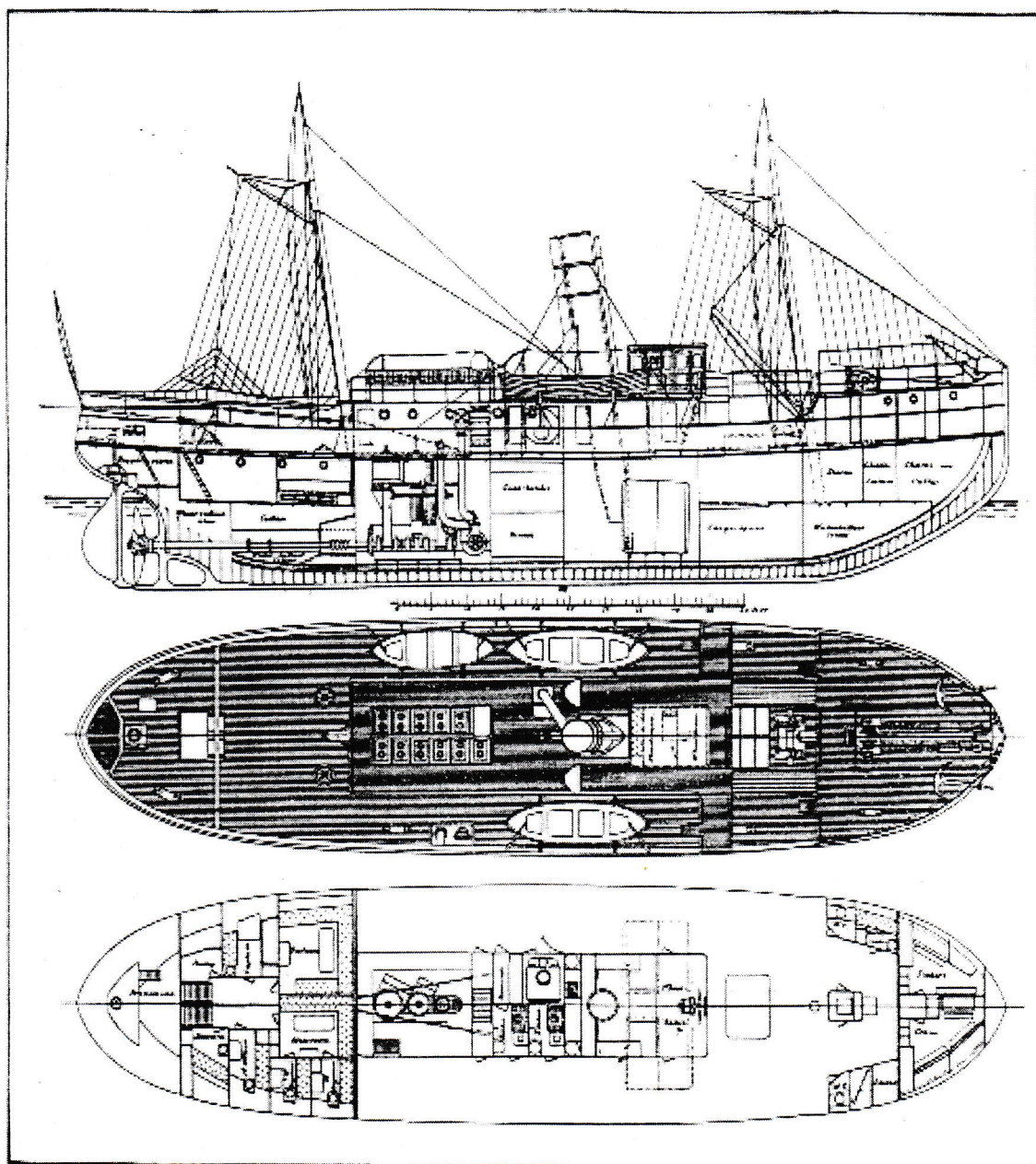
Projektritning för den ryska isbrytaren LEDOKOL, som enligt kontrakt av den 24 februari 1890 lät byggas på Lindholmens Varv i Göteborg s. å. för den Ryska Kejsarliga staten. Senare HOLMEN VIII (Åttan).
