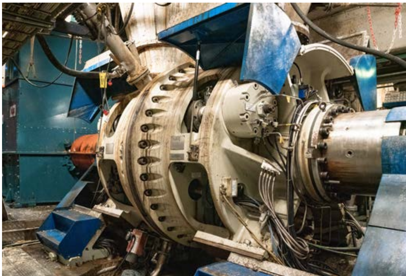
En av de två stora raffinörerna. Elförbrukningen för denna raffinör under en timme motsvarar elförbrukningen under ett helt år i en vanlig villa. Det är lätt att förstå att elpriset får stor betydelse för produktionskostnaden.
